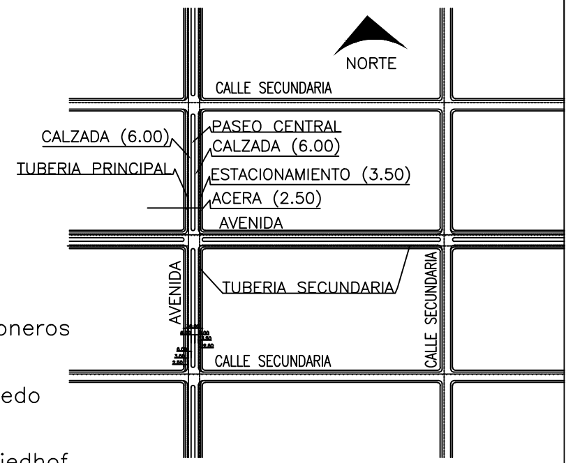
DETALLE DE UBICACIÓN DE TUBERIAS ORIENTACIÓN: NORTE - NOR OESTE SN ESCALA
